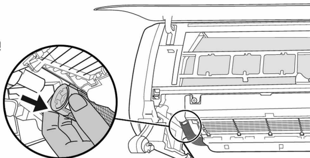
Biały węz odpływu skroplin
