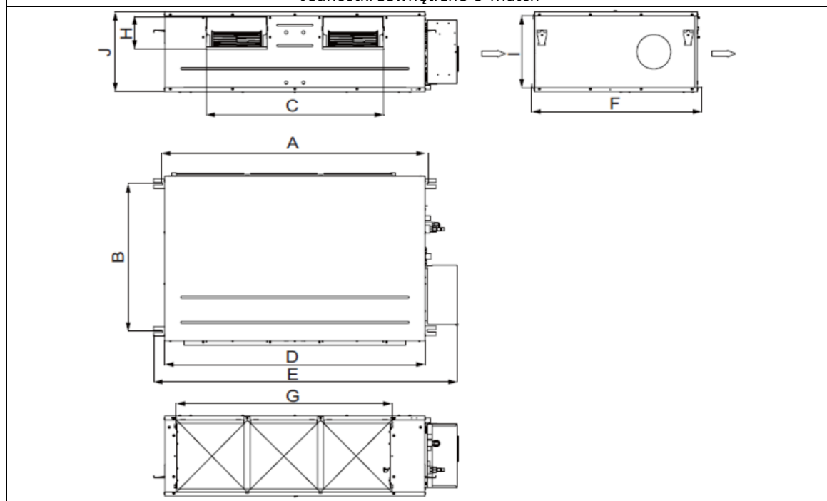
Jednostki wewnętrzne kanałowe
